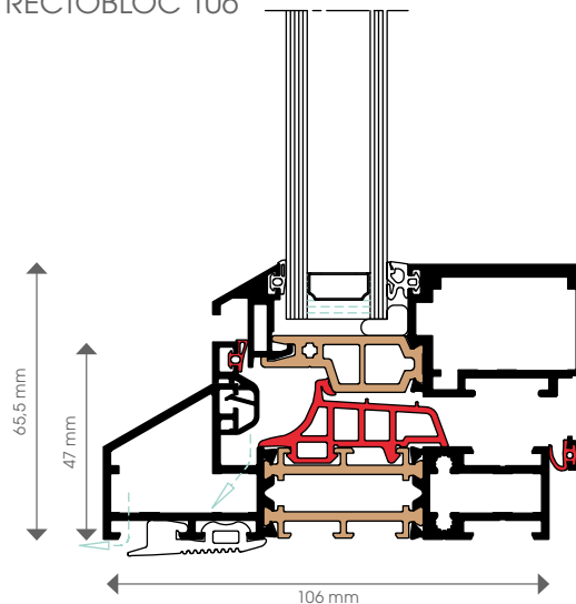
RECTOBLOC 106
