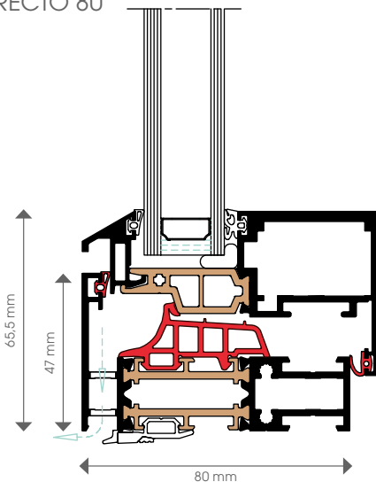
RECTO 80
